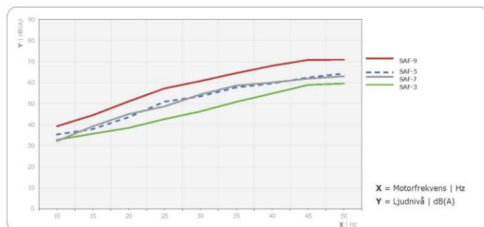
LJUDNIVÅ
