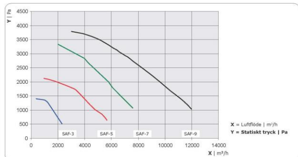
FLÄKTKURVOR
